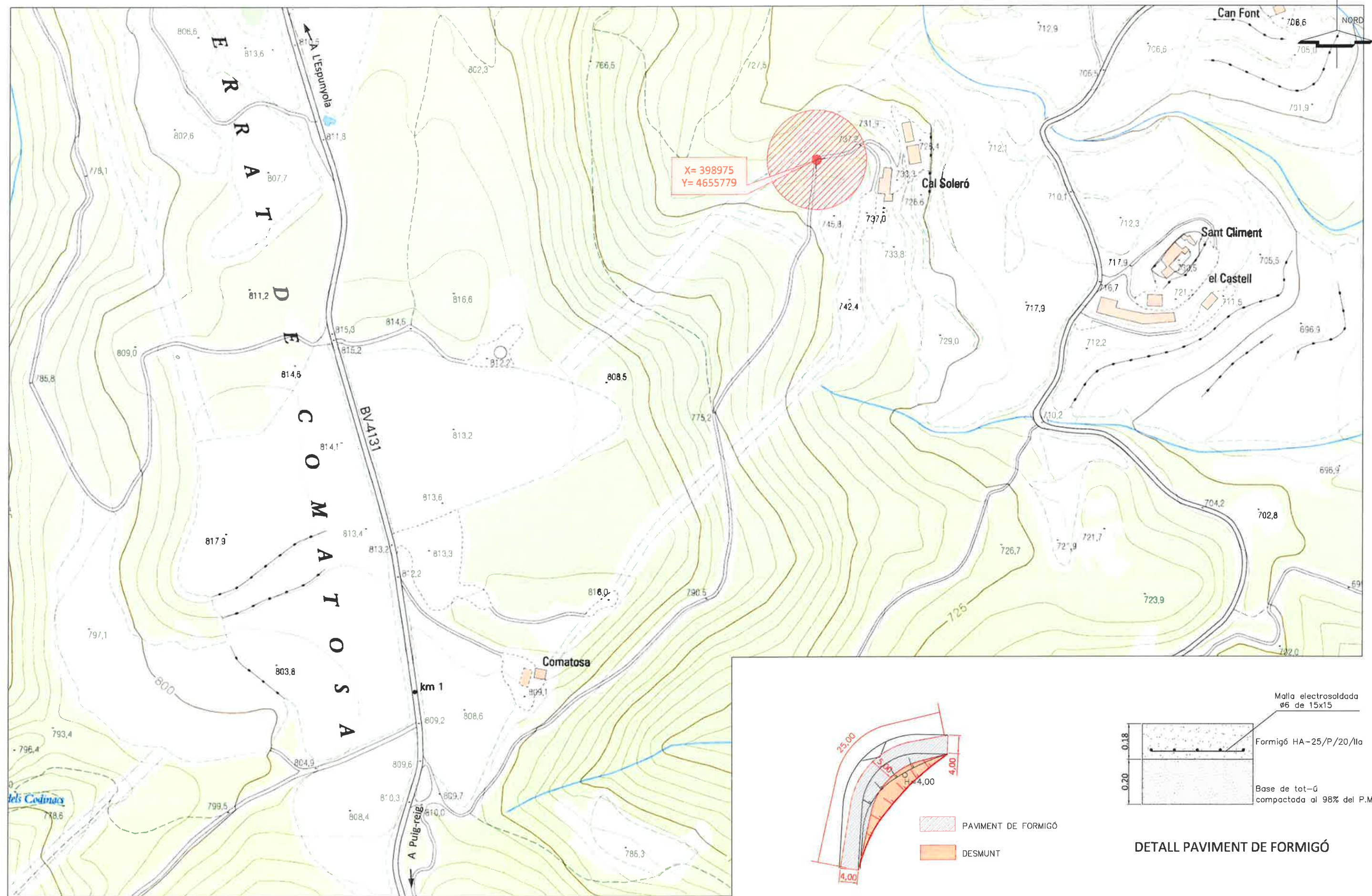
CROQUIS PLANTA
