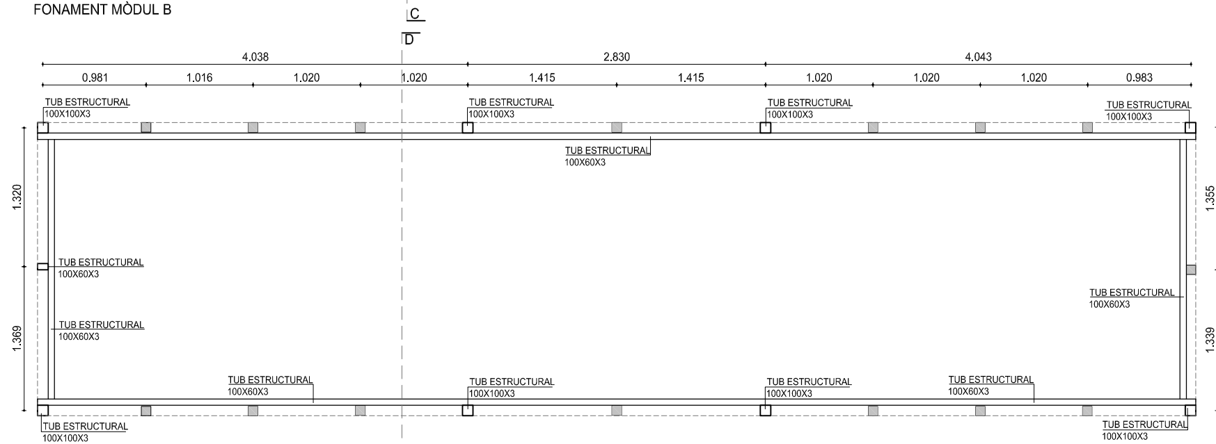
ESTRUCTURA COBERTA MÒDUL B
