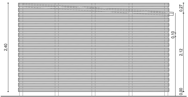
ECOPUNT. ALÇAT TRANSVERSAL POSTERIOR
