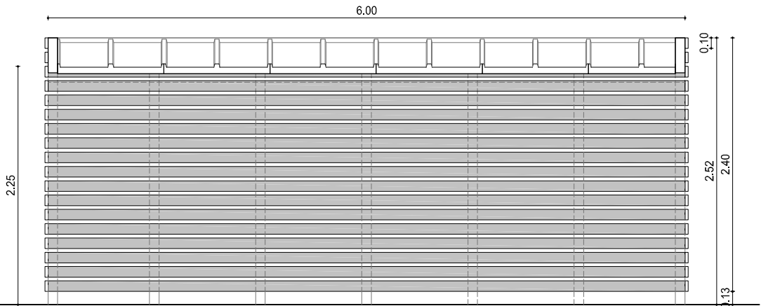
ECOPUNT. ALÇAT LONGITUDINAL COBERTA
