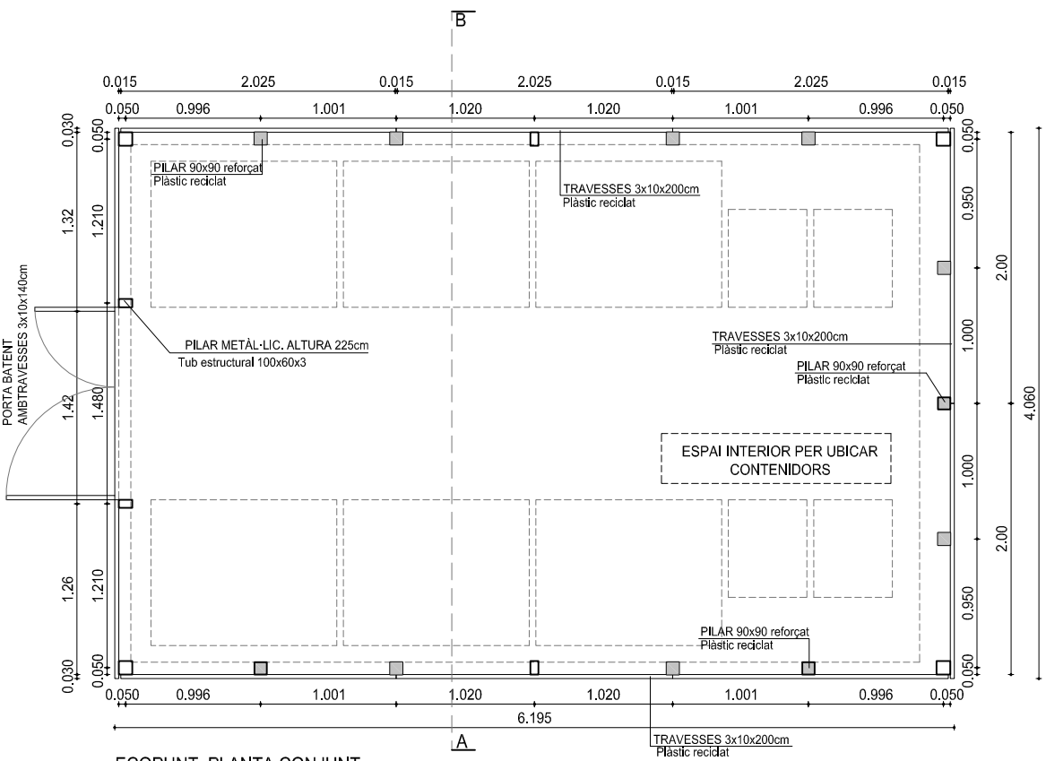
ECOPUNT. PLANTA CONJUNT
