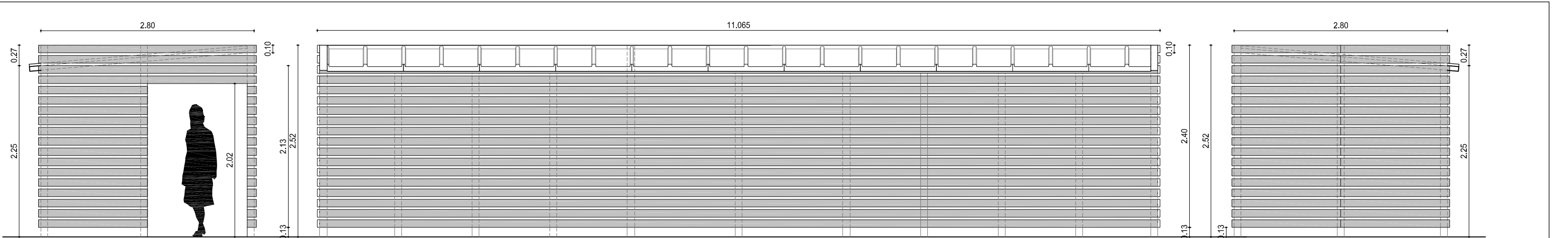
ECOPUNT. ALÇAT TRANSVERSAL
